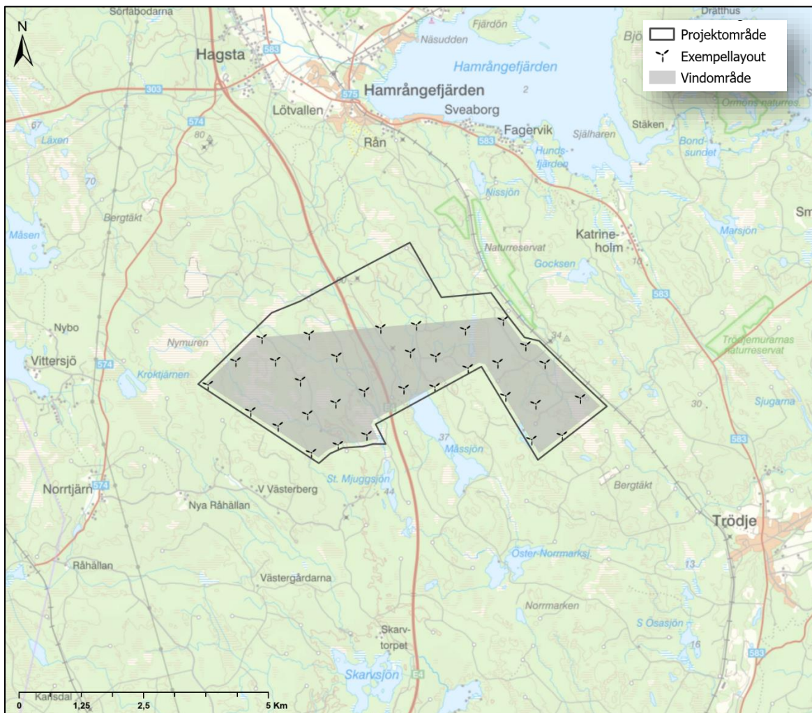
Figur 5. Utformningsexempel för Måssjöns Vindpark med 32 vindkraftverk. Datakälla: Bolaget.
