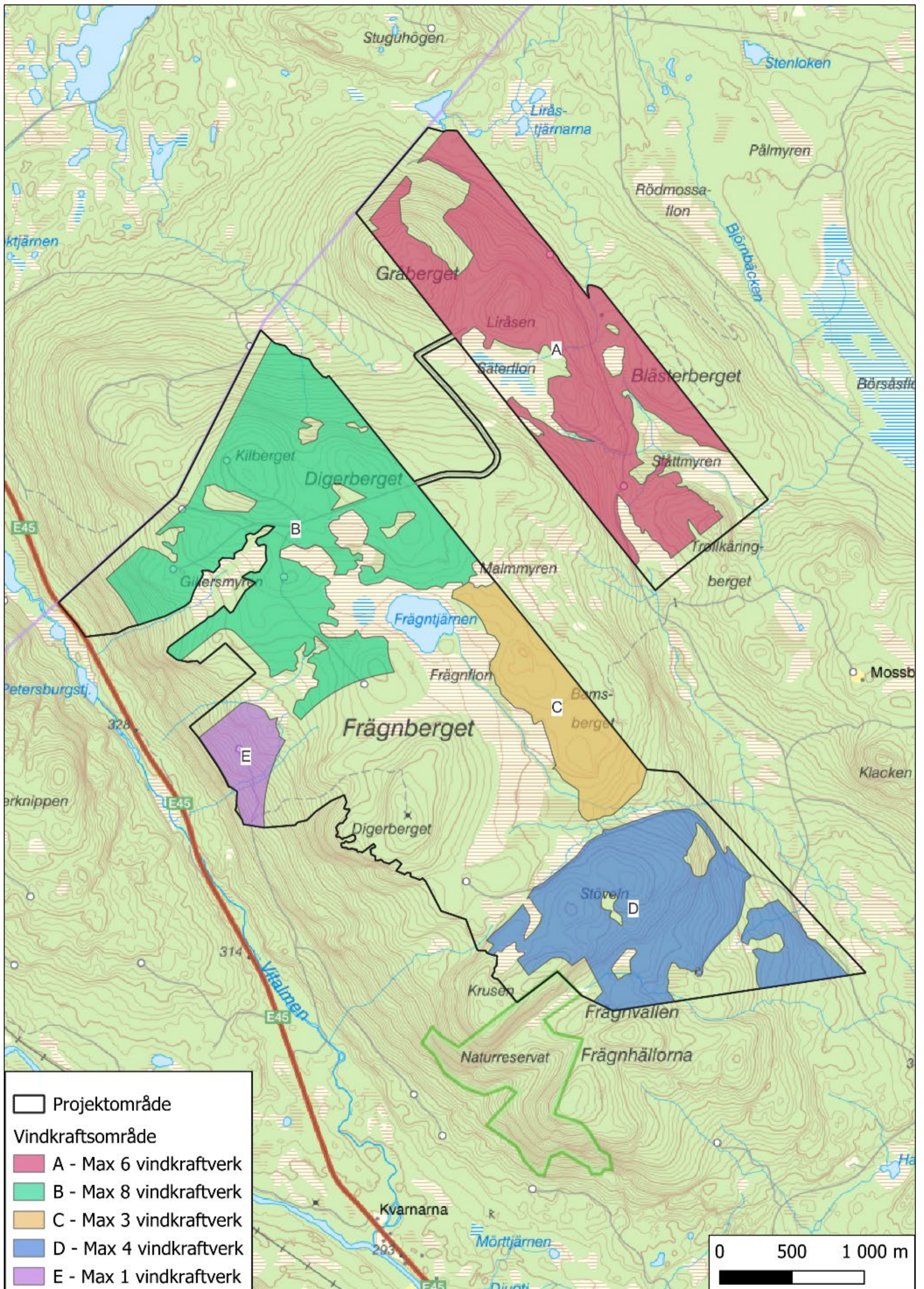
Figur 2. Ansökt utformning - Vindkraftsområden
