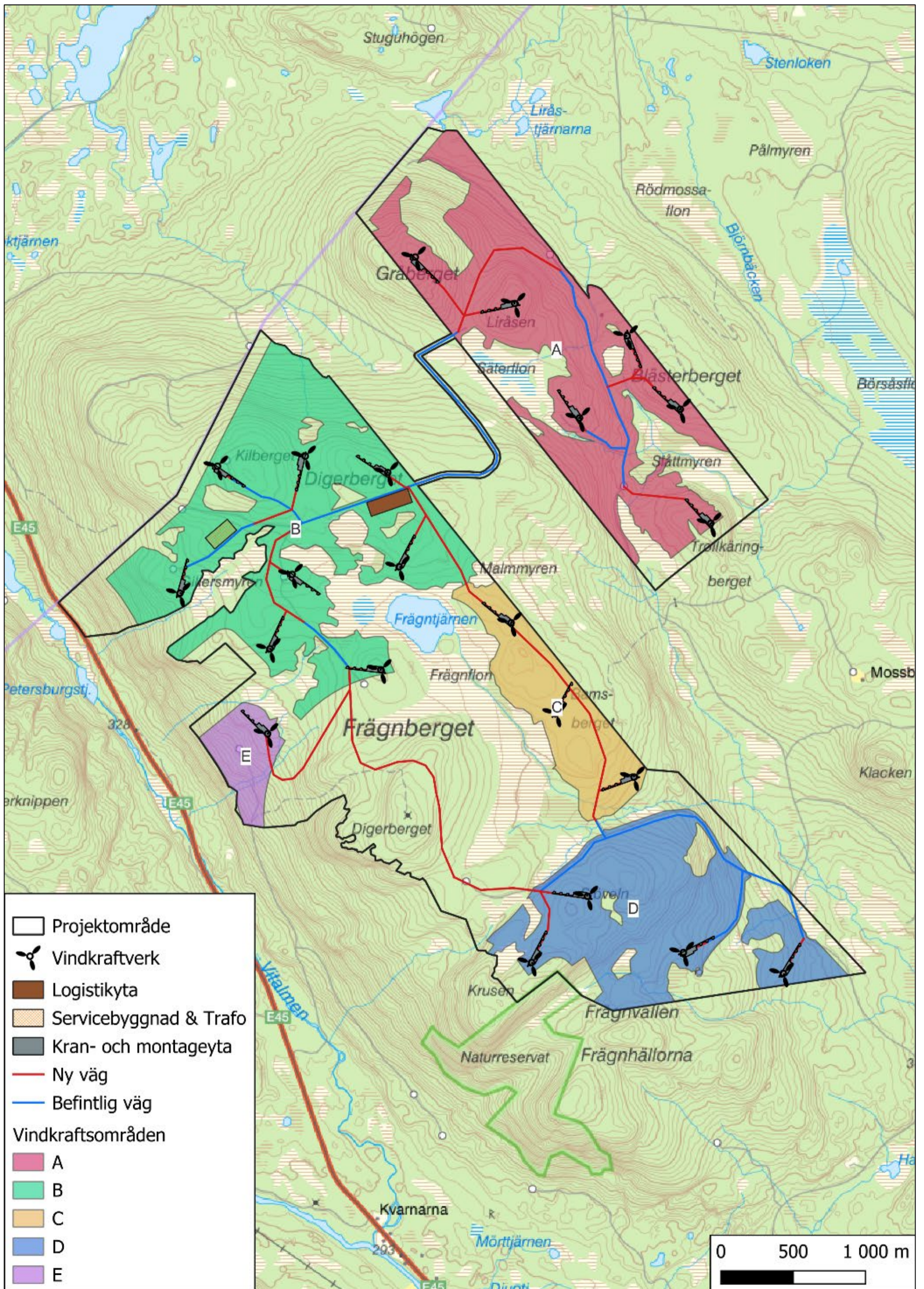
Figur 12. Exempelutformning med möjlig vägdragning samt övriga hårdgjorda ytor
