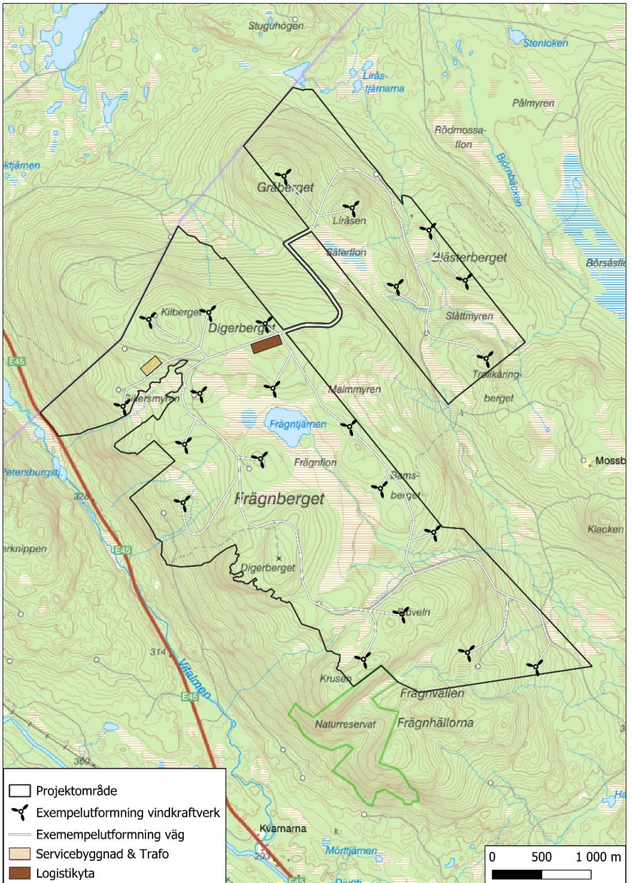
Figur 4. Exempelutformning med 22 vindkraftverk, servicebyggnad, transformatorstation, vägar samt tillfällig logistikyta
